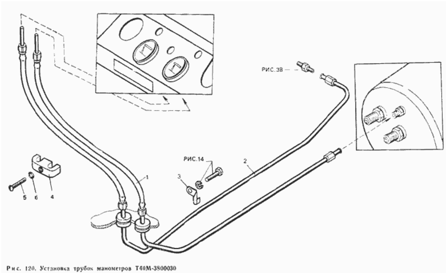
Рис. 120. Установка трубок манометров Т40М-3800030.
